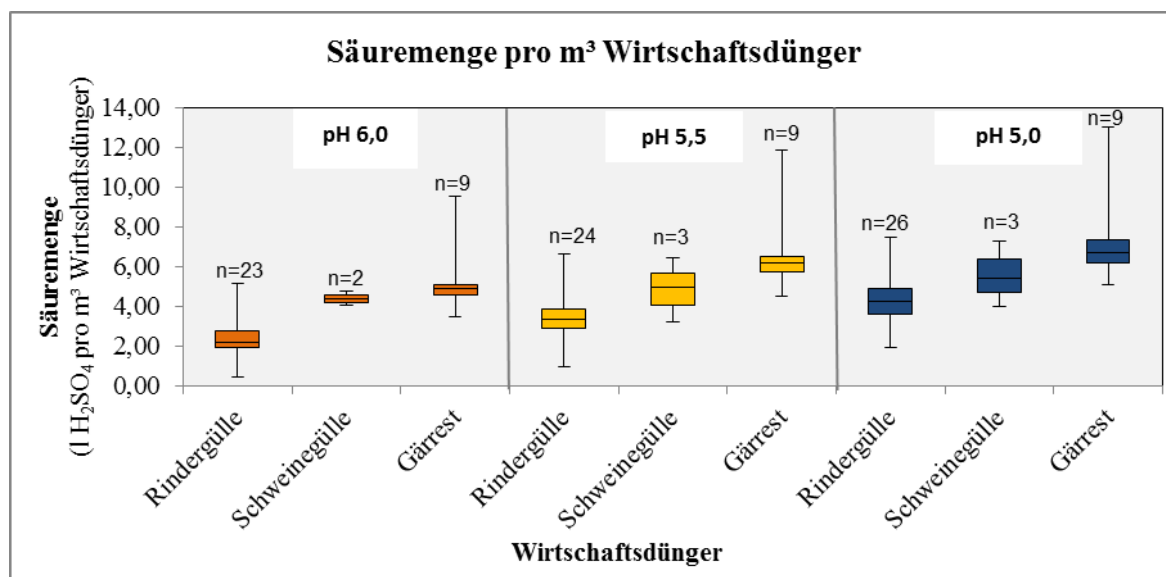
Benötigte Säuremenge pro m 3 Wirtschaftsdünger für eine pH-Wert-Absenkung auf pH 6, 5,5 und 5.
