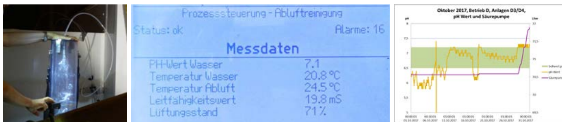
Probenahme Geruch (links), Anzeigemonitor neuer Filter (Mitte), Auswertung el. Betriebstagebuch (rechts)
