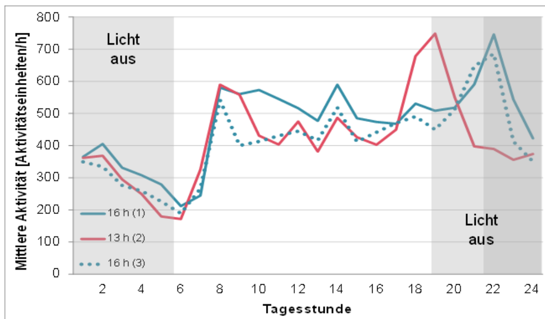
Mittlere Aktivität (in Aktivitätseinheiten/h) im Verlauf über 24 Stunden in den drei Versuchsphasen bei verschiedener Beleuchtungsdauer
