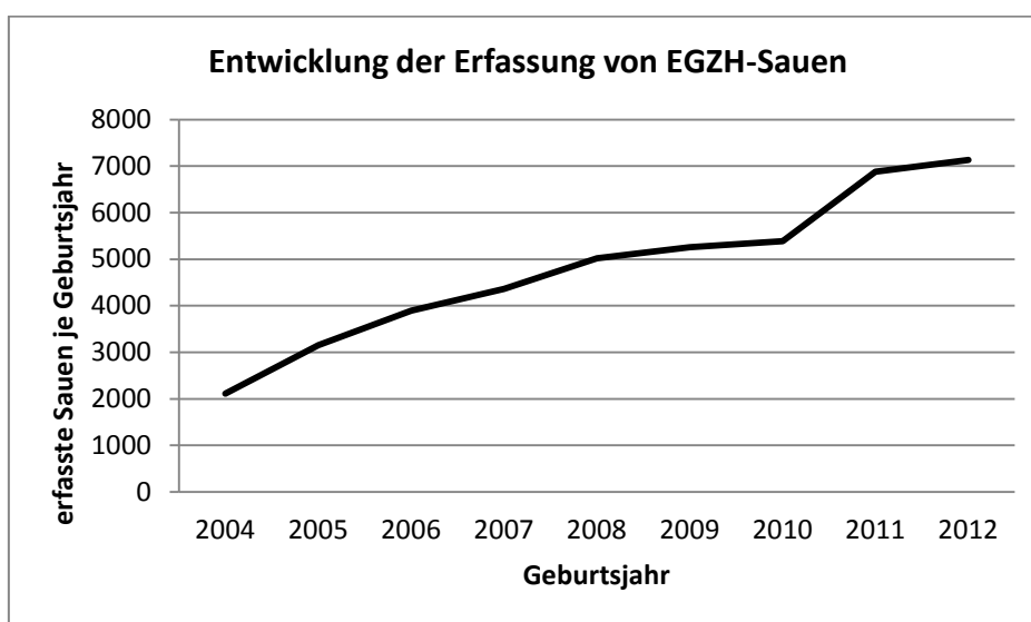
Abbildung 5: Entwicklung der im LKV-Sauenplaner erfassten EGZH-Jungsauen je Geburtsjahr
