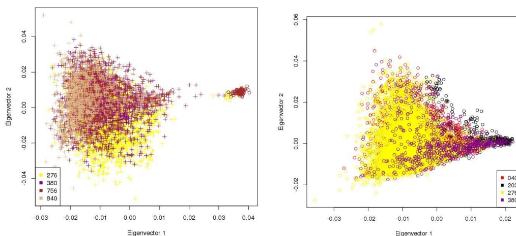
Abbildung 1: Ergebnisse erster Strukturanalysen, dargestellt sind standardisierte genetische Distanzen. Links: Ergebnisse der Rasse Braunvieh. Rechts: Ergebnisse der Rasse Fleckvieh. Verwendete Ländercodes: Deutschland (276), Österreich (040), Tschechien (203), Italien (380), Schweiz (756), USA (840).
