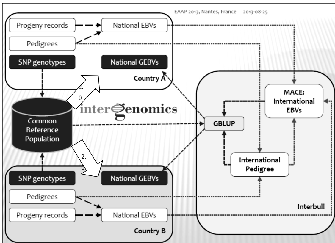
Abbildung 1: Schematischer Überblick zu InterGenomics (Duerr, EAAP Nantes, 2013) erweitert um die Rücklieferung aller Genotypen an die nationalen Rechenstellen im Rahmen von InterGenomics 2.0.
