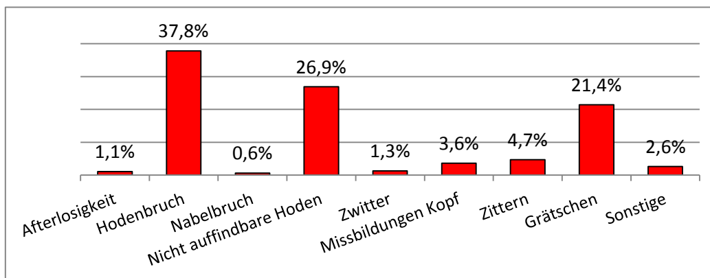
Abbildung 1: Verteilung der Anomalien bei den betroffenen Ferkeln
