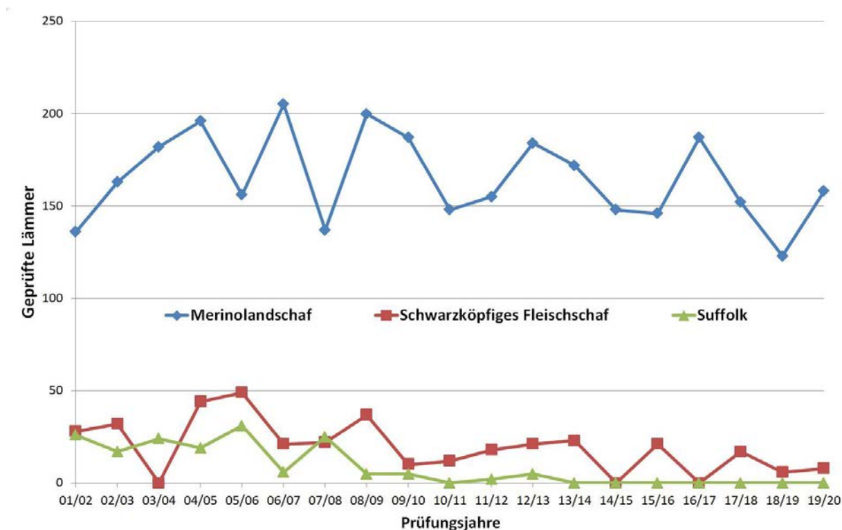
Abbildung 1: Anzahl geprüfter Tiere der Jahrgänge 2001/02 bis 2019/20
